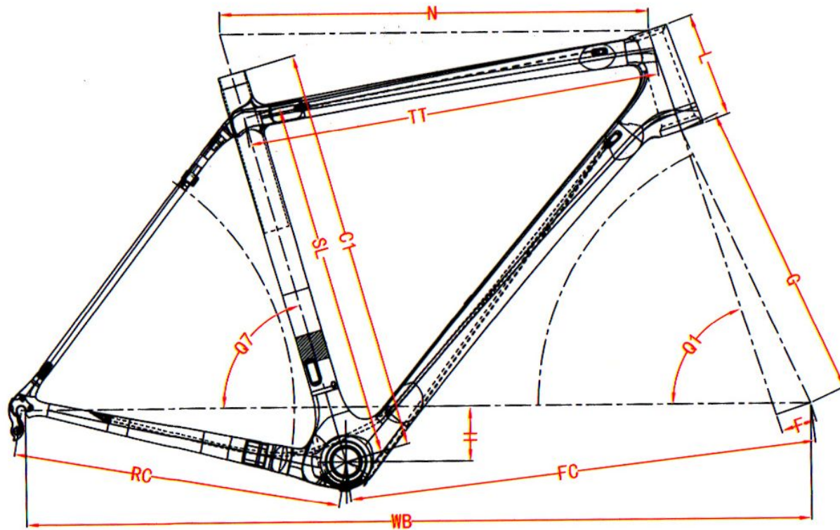
SFIDA Avventura ディスクブレーキ対応フレーム(SFIDA-300, JAN:4573415850011)
